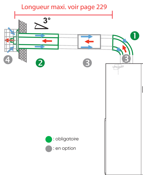
C Ventouse horizontale télescopique
