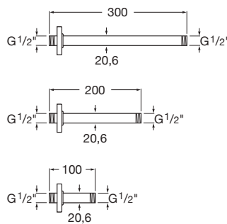
Bras mural carré pour pomme de douche. Compatible avec RainDream et RainSense.
