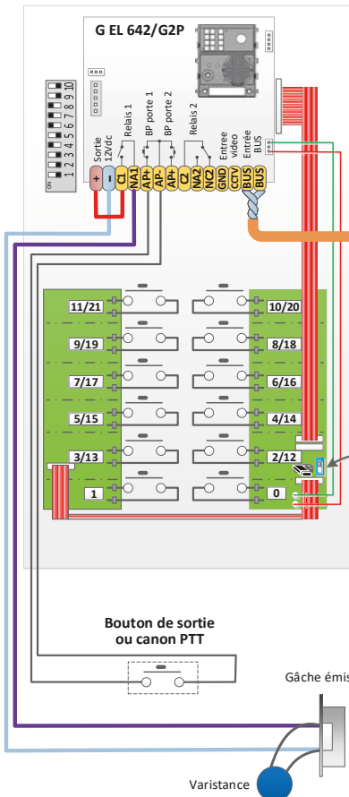
Câblage bouton Platine GTV62/ XXX
